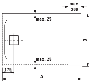
Shower tray, made-to-measure Duschwanne auf Maß 212950
